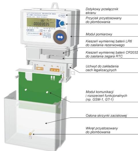
Budowa licznika LABM
