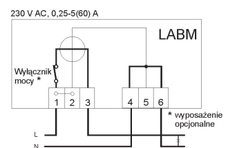
LABM z wyłącznikiem mocy
