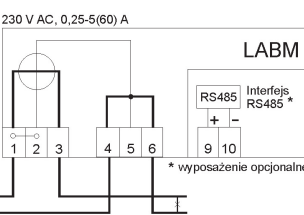
LABM z interfejsem RS485
