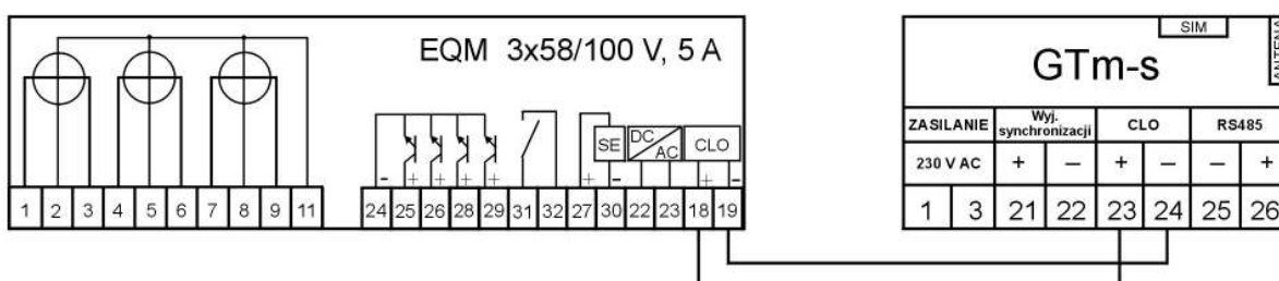
Rys. 4. Przykładowy schemat połączenia modułu komunikacyjnego GTm-s z licznikiem typu EQM (3x58/100 V, 5 A) wyposażonym w interfejs komunikacyjny CLO
