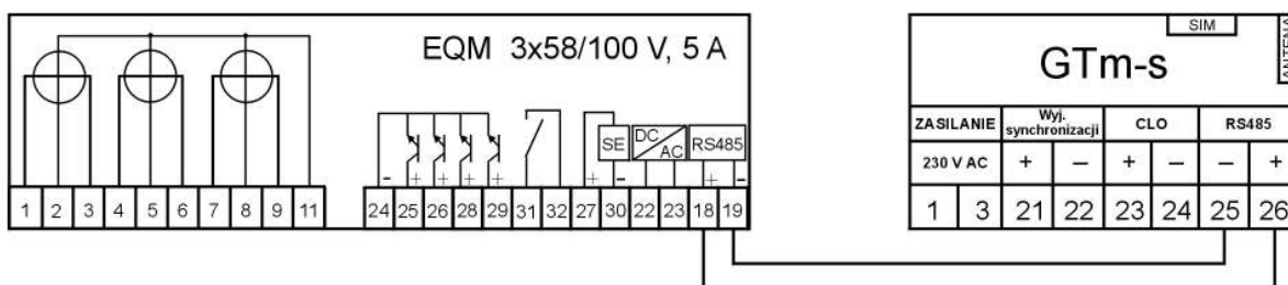
Rys. 3. Przykładowy schemat połączenia modułu komunikacyjnego GTm-s z licznikiem typu EQM (3x58/100 V, 5 A) wyposażonym w interfejs komunikacyjny RS485
