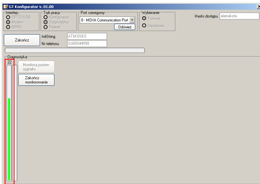
Rys. 21. Diagnostyka przez modem (dla połączenia w trybie CSD)
