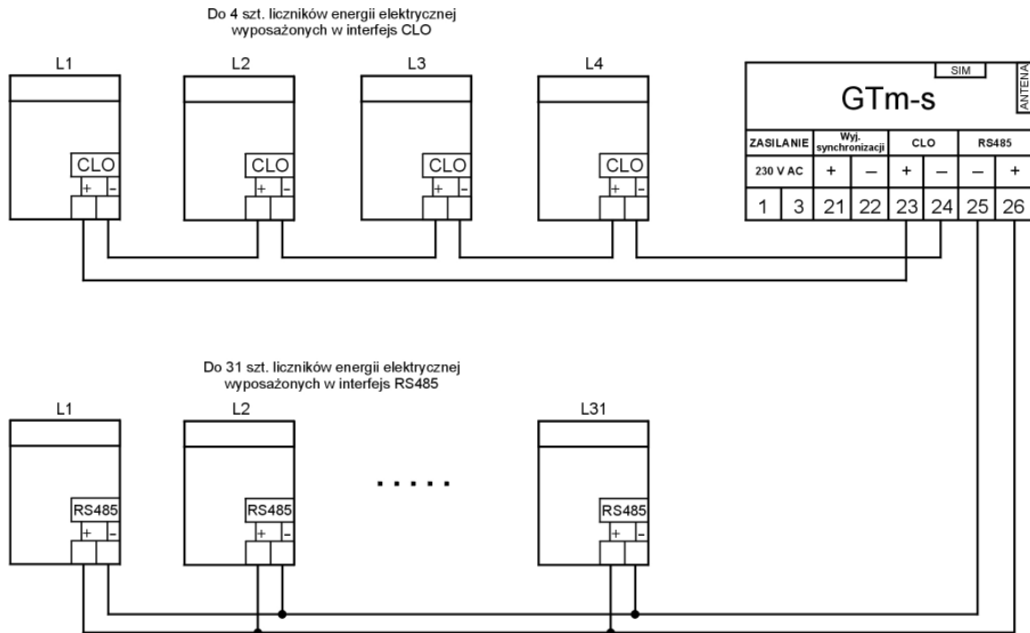
Rys. 7. Przykładowy schemat połączenia modułu komunikacyjnego GTm-s z licznikami wyposażonymi w interfejs komunikacyjny pętli prądowej CLO oraz RS485
