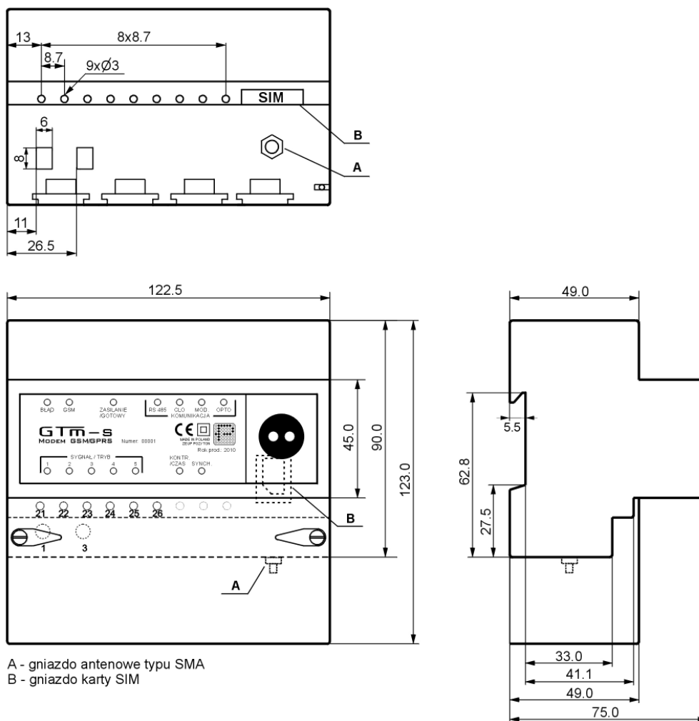
Rys. 1. Wymiary modułu komunikacyjnego GTm-s
