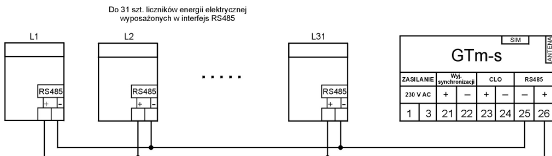
Rys. 5. Przykładowy schemat połączenia modułu komunikacyjnego GTm-s z licznikami wyposażonymi w interfejs komunikacyjny RS485
