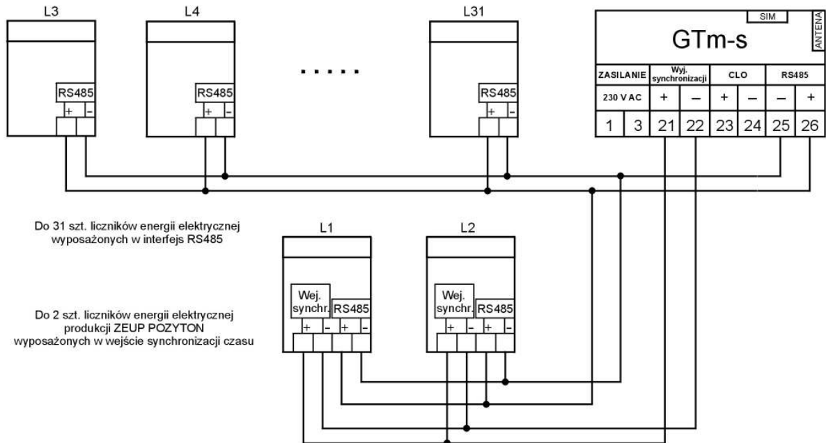
Rys. 8. Przykładowy schemat połączenia modułu komunikacyjnego GTm-s z wykorzystaniem funkcji synchronizacji czasu zegara RTC liczników energii elektrycznej produkcji ZEUP Pozyton
