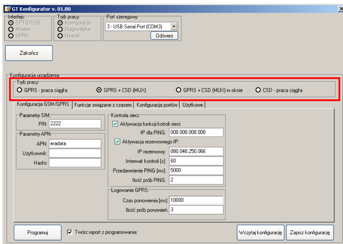
Rys. 13. Wybór trybu pracy modułu komunikacyjnego GTm-s
