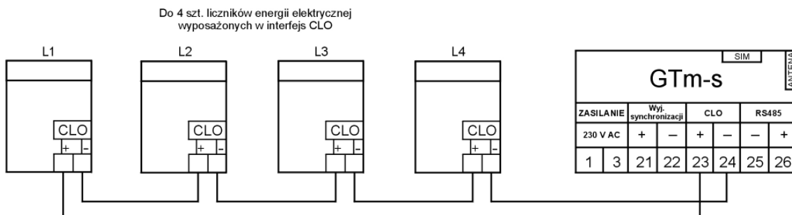
Rys. 6. Przykładowy schemat połączenia modułu komunikacyjnego GTm-s z licznikami wyposażonymi w interfejs komunikacyjny pętli prądowej CLO
