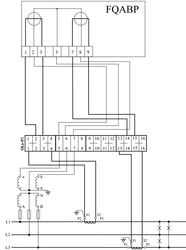
Licznik FQABP 3x100 V, 5 A
